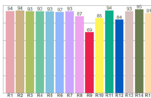
CRI: 92.4 (R1-R8)
